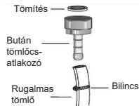
Rugalmas tömlő
