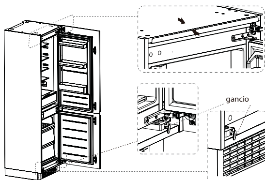
Piegatura del bordo del deflettore superiore
