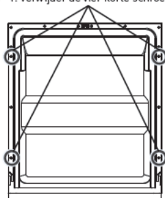
B 1. Verwijder de vier korte schroeven
